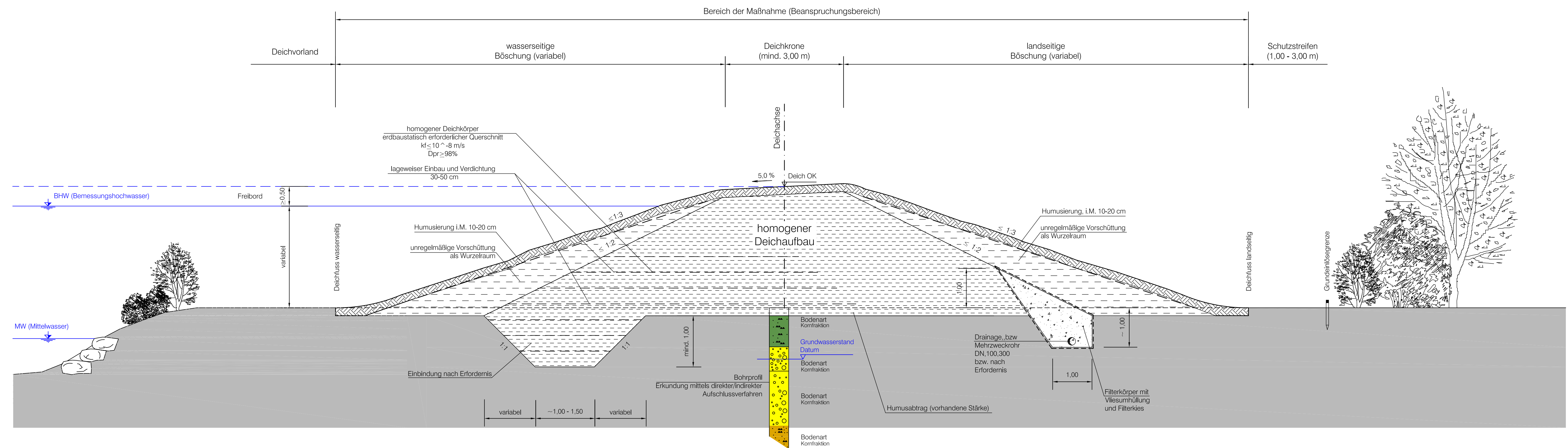
Musterdeich, empfohlener Querschnitt, homogener Deichkörper
