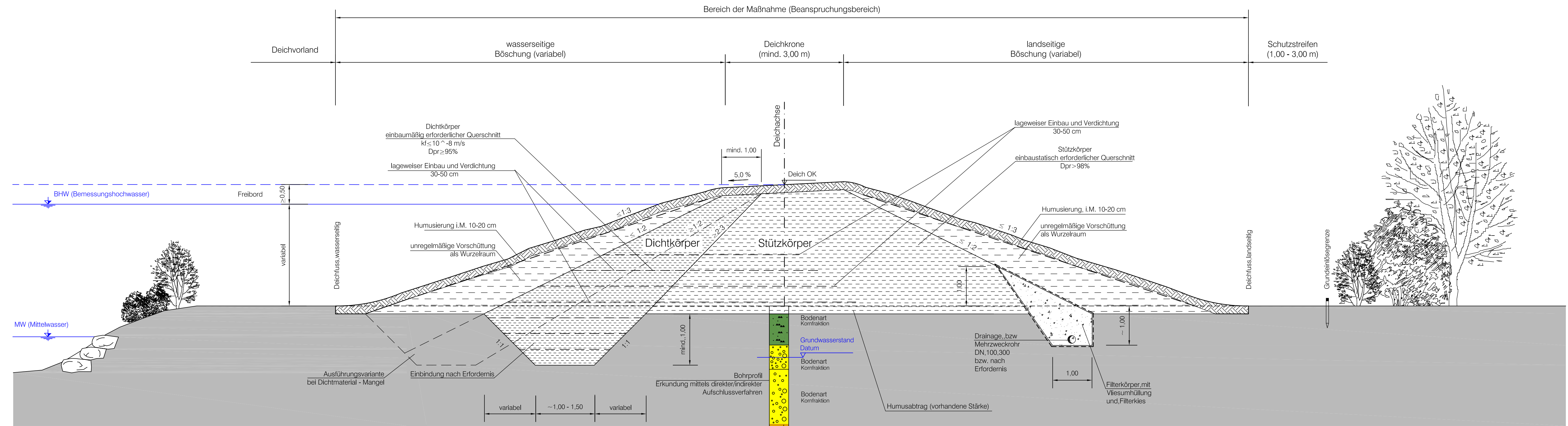
Musterdeich, empfohlener Querschnitt, zonierter Deichkörper
