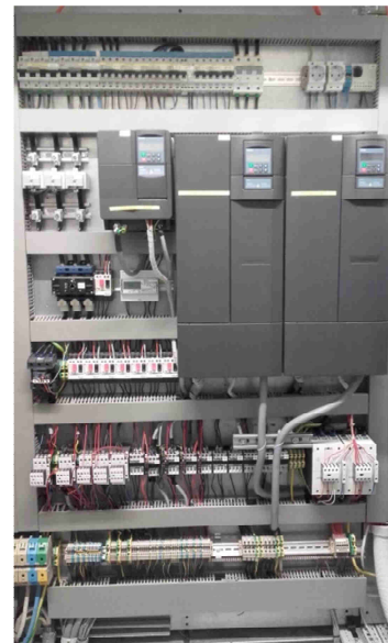
Schaltkasten
