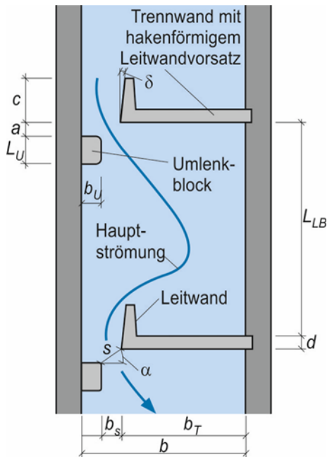
Abbildung 33 Geometrische Kennwerte eines Schlitzpasses DWA –Merkblatt M509 (2014)
