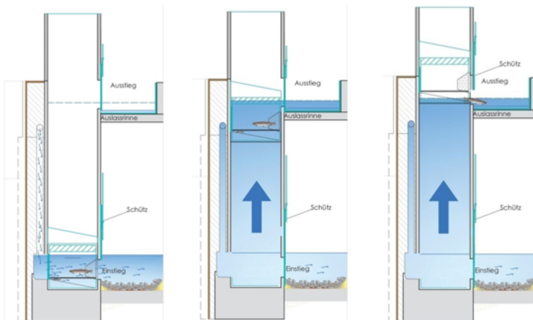
Abbildung 60 Betriebsweise des kombinierten Fischlifftsystems (links: Einschwimmphase, Mitte: Hub, rechts: Ausstiegsphase)
