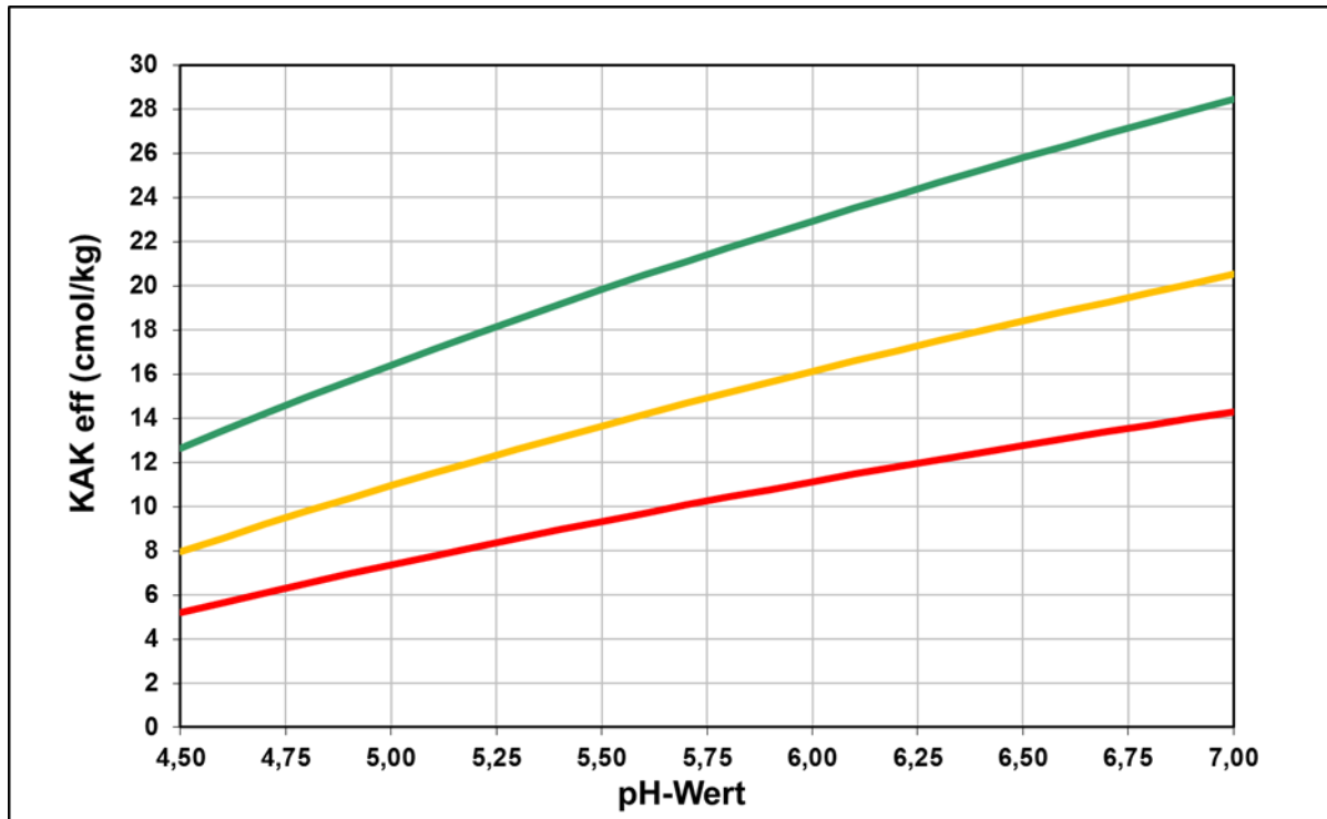
Abbildung 6: pH-Wert und effektive KAK von leichten (Ton < 15 %, Humus < 2,5 %: rote Linie), mittleren (Ton 15-25 %, Humus 2,53,75 %: gelbe Linie) und schweren Böden (Ton > 25 %, Humus 2,56,5 %: grüne Linie)
