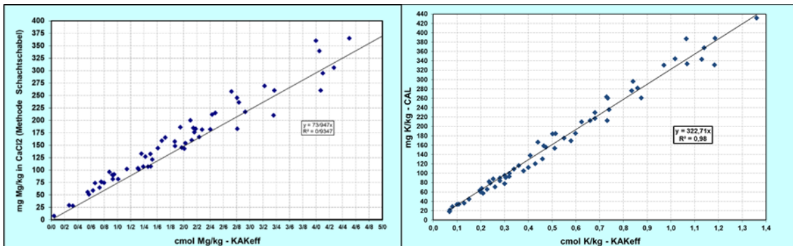
Abbildung 10: Zusammenhang zwischen austauschbarem Kalium und Magnesium (KAK eff ) und dem „pflanzenverfügbaren“ Kalium (K-CAL) und Magnesium (in CaCl 2 ): 63 Datensätze aus ALVA-Ringversuchen aus den Jahren 2000 - 2020 (je 3 Proben pro Jahr)
