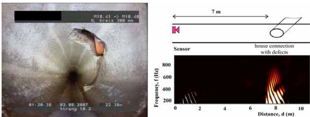
Abbildung 198 - TV-Befahrung vs. SewerBatt® Inspektionsergebnisse - Zustandsgruppen (Plihal et al., 2015)
