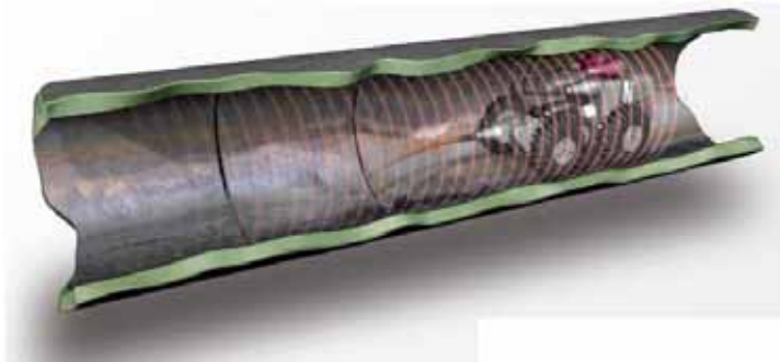
Abbildung 14 - Laser Profiler Funktionsweise (Hartl, 2009)
