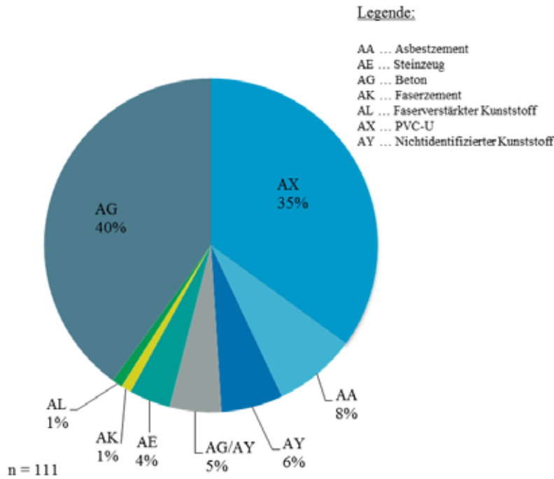
Abbildung 39 - Felduntersuchungen in Kombination Elektronischer Spiegel und SewerBatt® - Haltungsmaterialien
