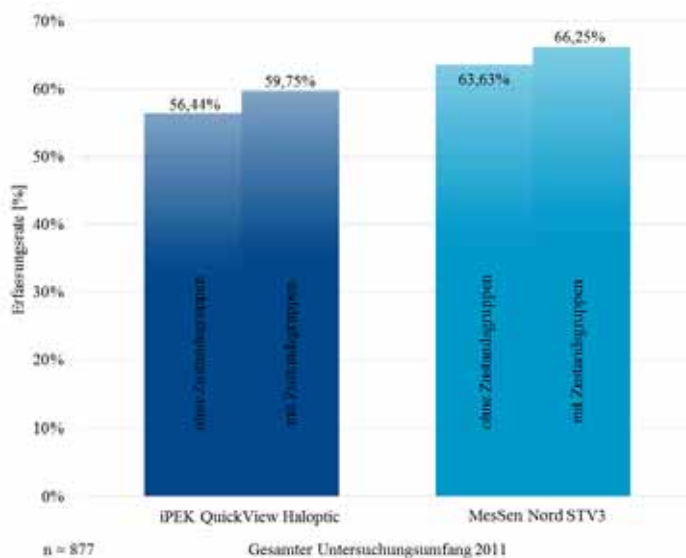
Abbildung 137 - Änderung der Erfassungsraten der elektronischen Spiegelmodelle bei Anwendung von Zustandsgruppen Untersuchungsumfang 2011
