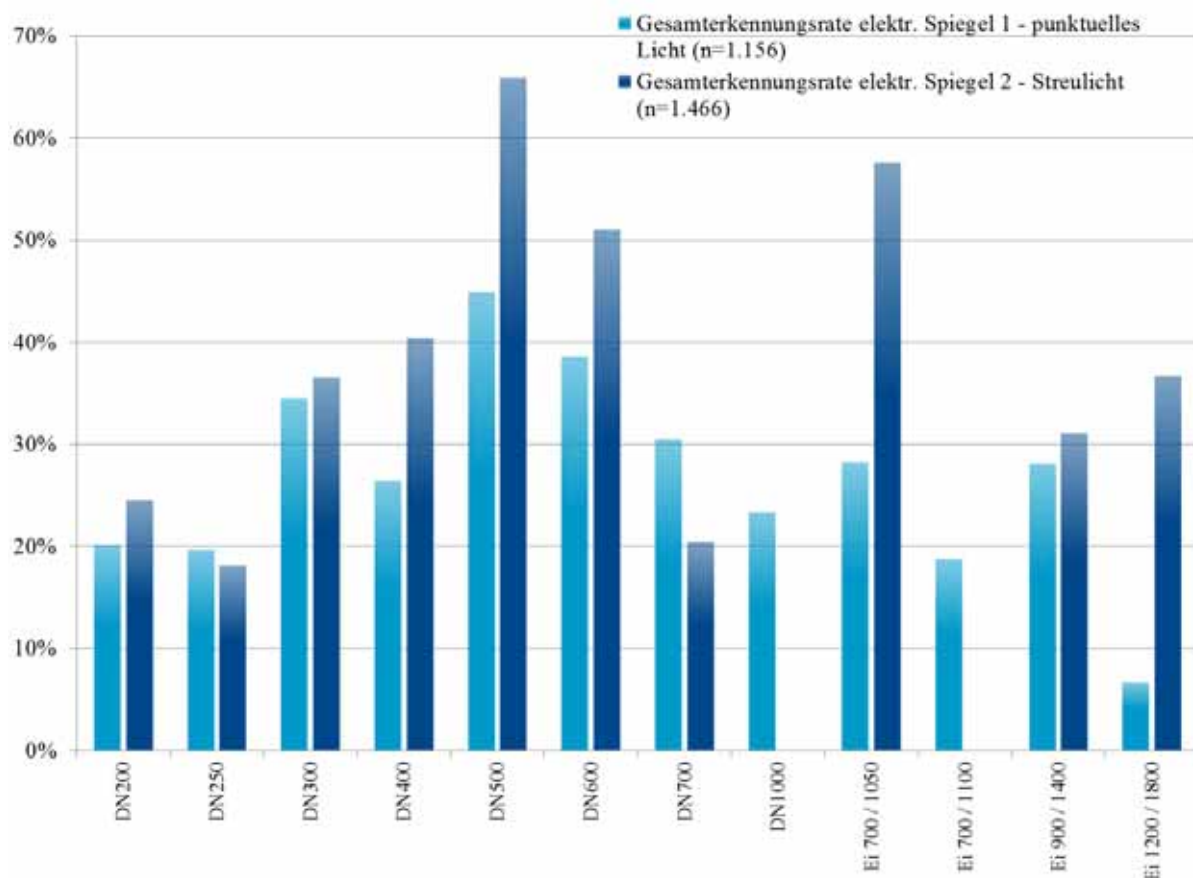
Abbildung 82 - Zustandserkennungsraten in verschiedenen Haltungsdimensionen
