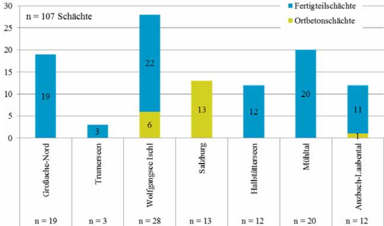
Abbildung 41 – Untersuchungsumfang Ortbetonschächte/Fertigteilschächte
