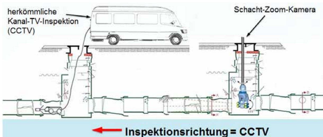
Abbildung 11 - Elektronischer Spiegel: Gleiche Inspektionsrichtung wie herkömmliche TV-Inspektion (adaptiert nach Aquadata, 2012)
