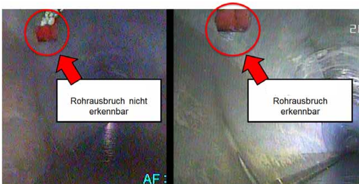
Abbildung 103 - Vergleich unterschiedlicher Kameraauflösungen beim elektronischen Spiegel
