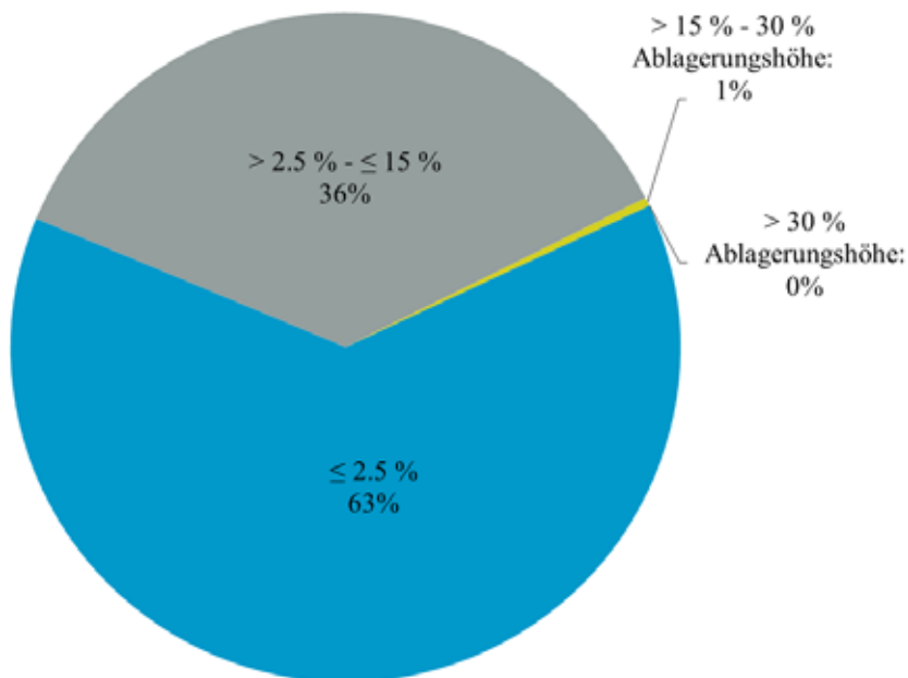
Abbildung 146 - Anteile Ablagerungshöhe in Haltungen der Mischwasserkanalisation
