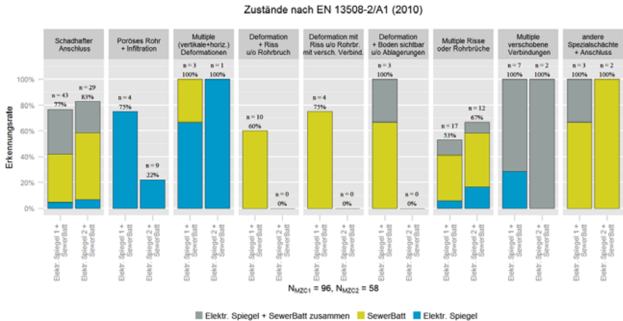
Abbildung 108 - Felduntersuchungen - Erkennungsraten für gruppierte Zustände und kombinierte Inspektionsgeräte (Plihal et al., 2015)
