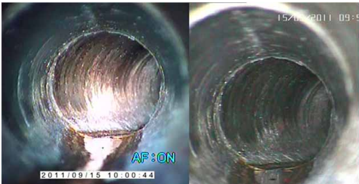
Abbildung 31 - Sicht bis zum Endschacht nicht möglich - zu große Abwinkelung in der Haltung
