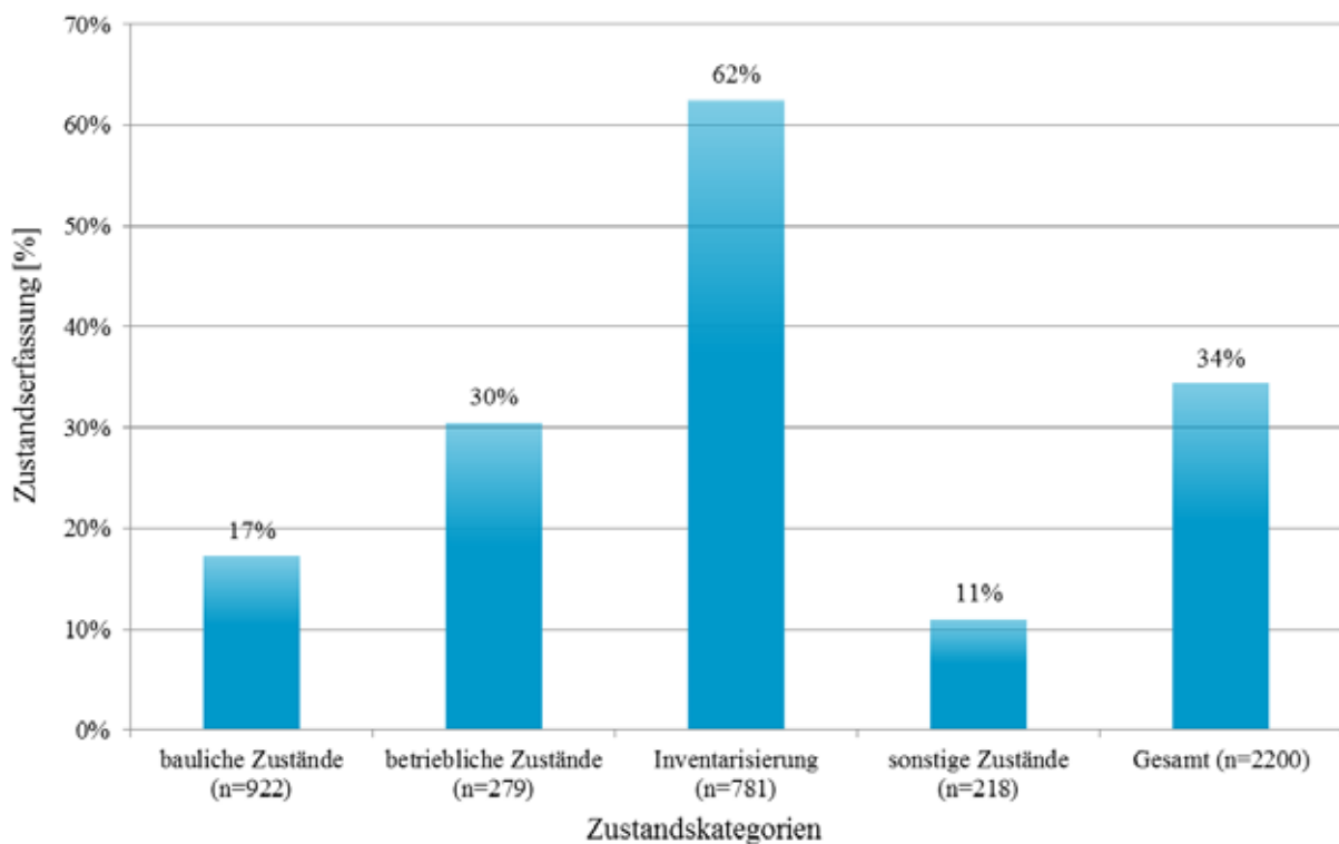
Abbildung 126 - Zustandserfassung elektronischer Spiegel ohne Zustandsgruppen 2009/10/12
