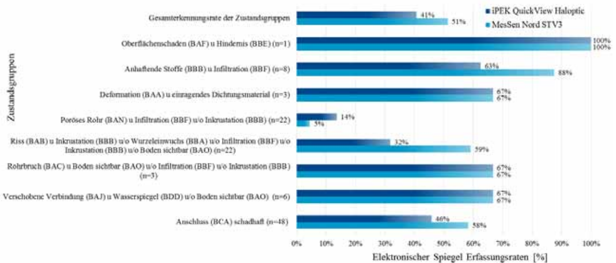
Abbildung 135 - Zustandserfassung der Zustandsgruppen mit den elektronischen Spiegelmodellen 2011
