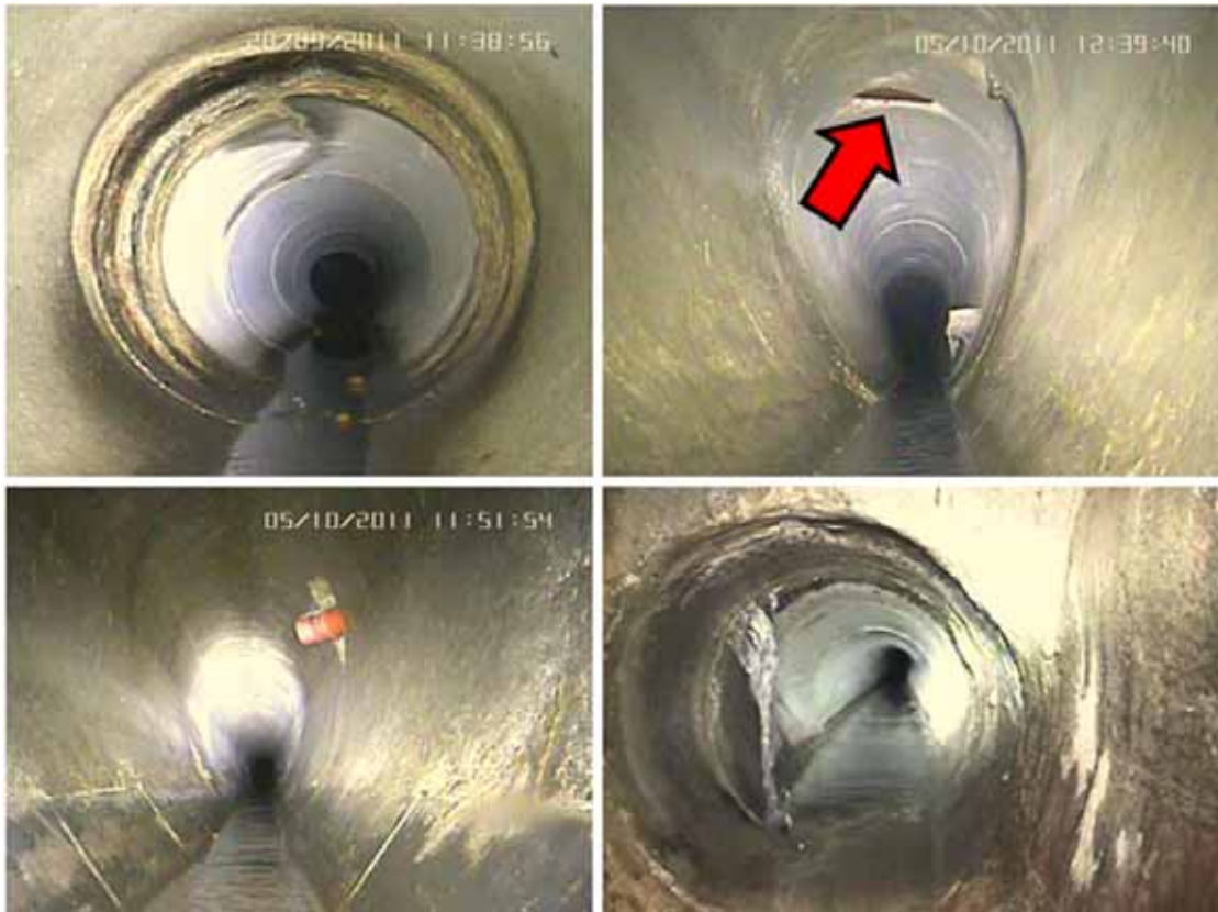
Abbildung 84 - Haltungen mit zusätzlichem Inspektionsbedarf
