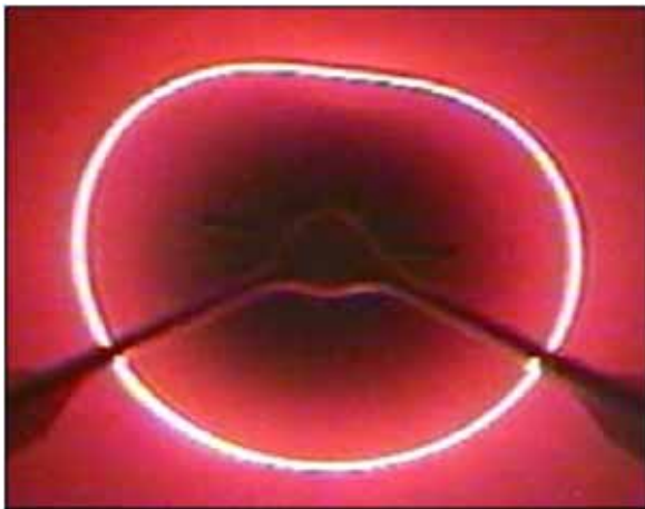
Abbildung 17 - TV-Ansicht während der Laser Profiler Vermessung (Hartl, 2009)
