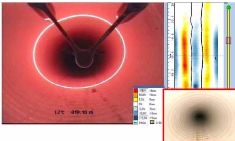
Abbildung 77 - Laser Profiler - Beispiel einer Aufnahme mit 15%iger Deformation (PE DN 200)
