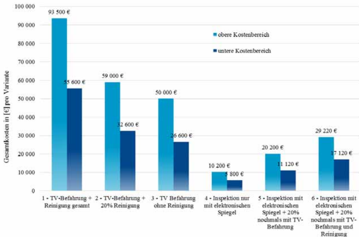
Abbildung 212 - Kosten für Varianten der Inspektion (und Reinigung) eines 20km langen Kanalisationsnetzes (Kuratko, 2015)
