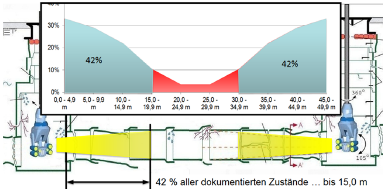
Abbildung 79 - Haltungsinspektion mit dem elektronischem Spiegel (adaptiert nach Aquadata, 2012)
