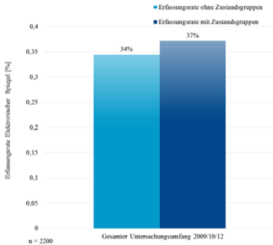
Abbildung 136 - Änderung der Erfassungsraten des elektronischen Spiegels bei Anwendung von Zustandsgruppen Untersuchungsumfang 2009/10/12
