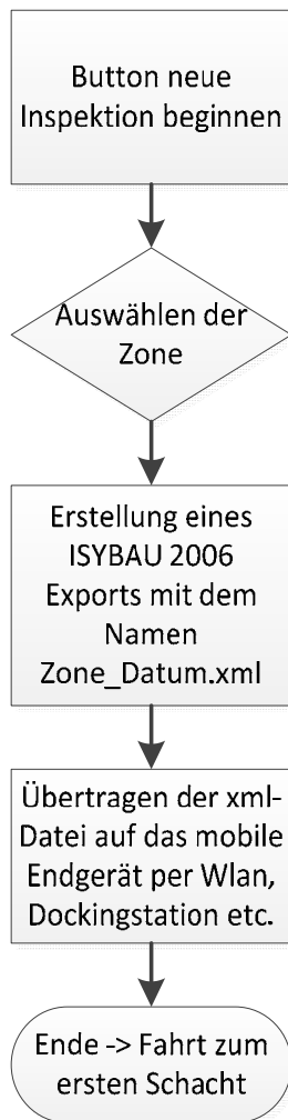
Abbildung 153 - Use-Case Inspektionsbeginn
