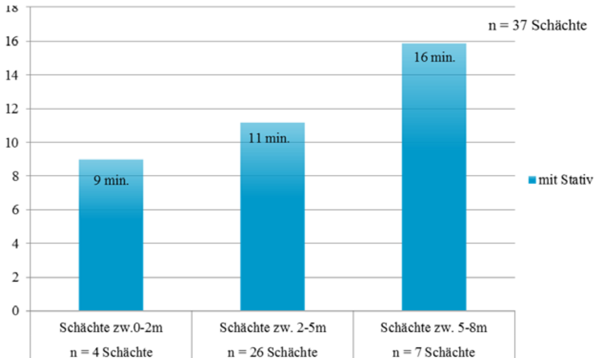
Abbildung 119 - Durchschnittliche Inspektionszeit pro Schacht mit Stativ
