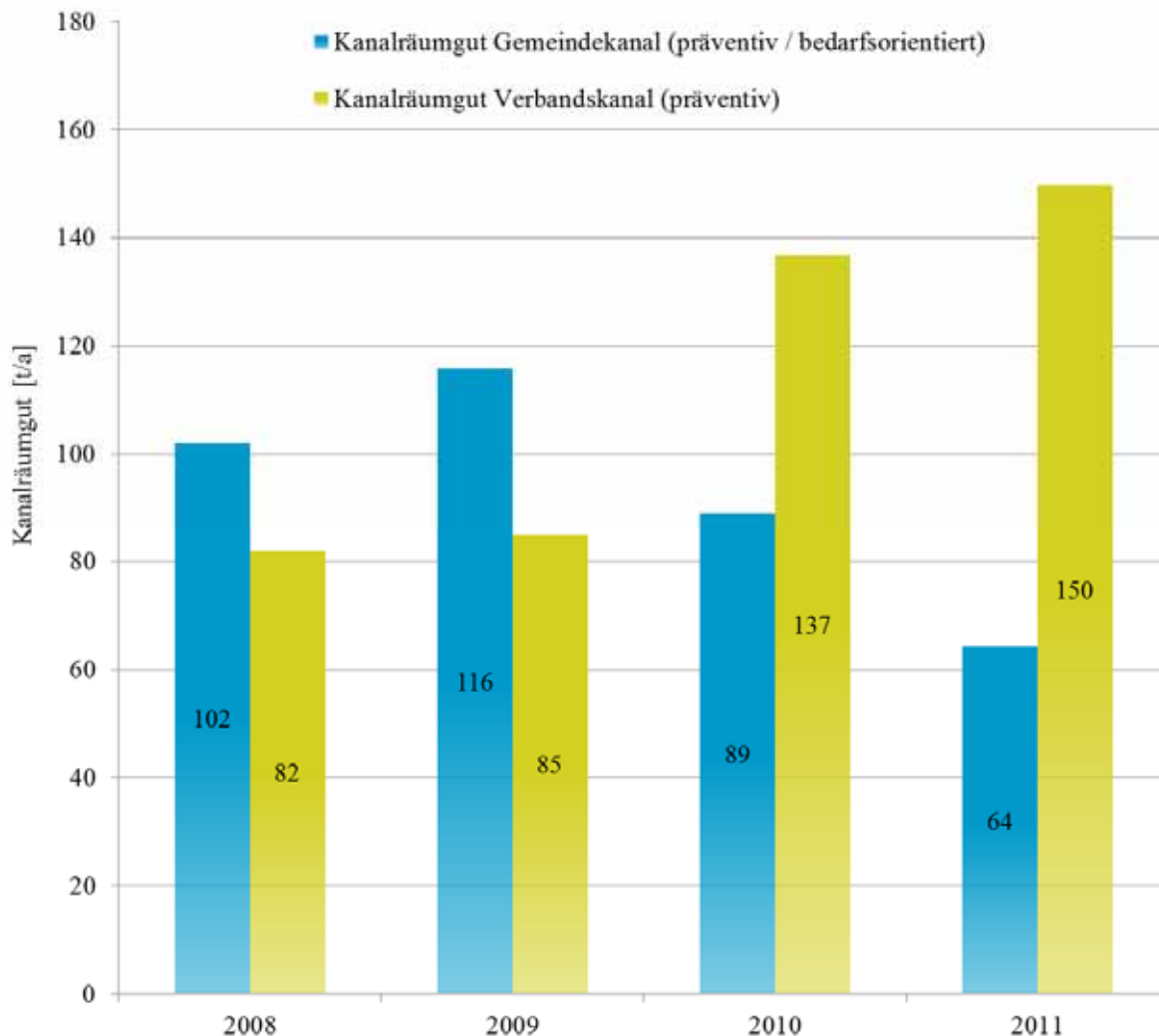
Abbildung 149 - Auswirkungen der geänderten Reinigungsstrategie
