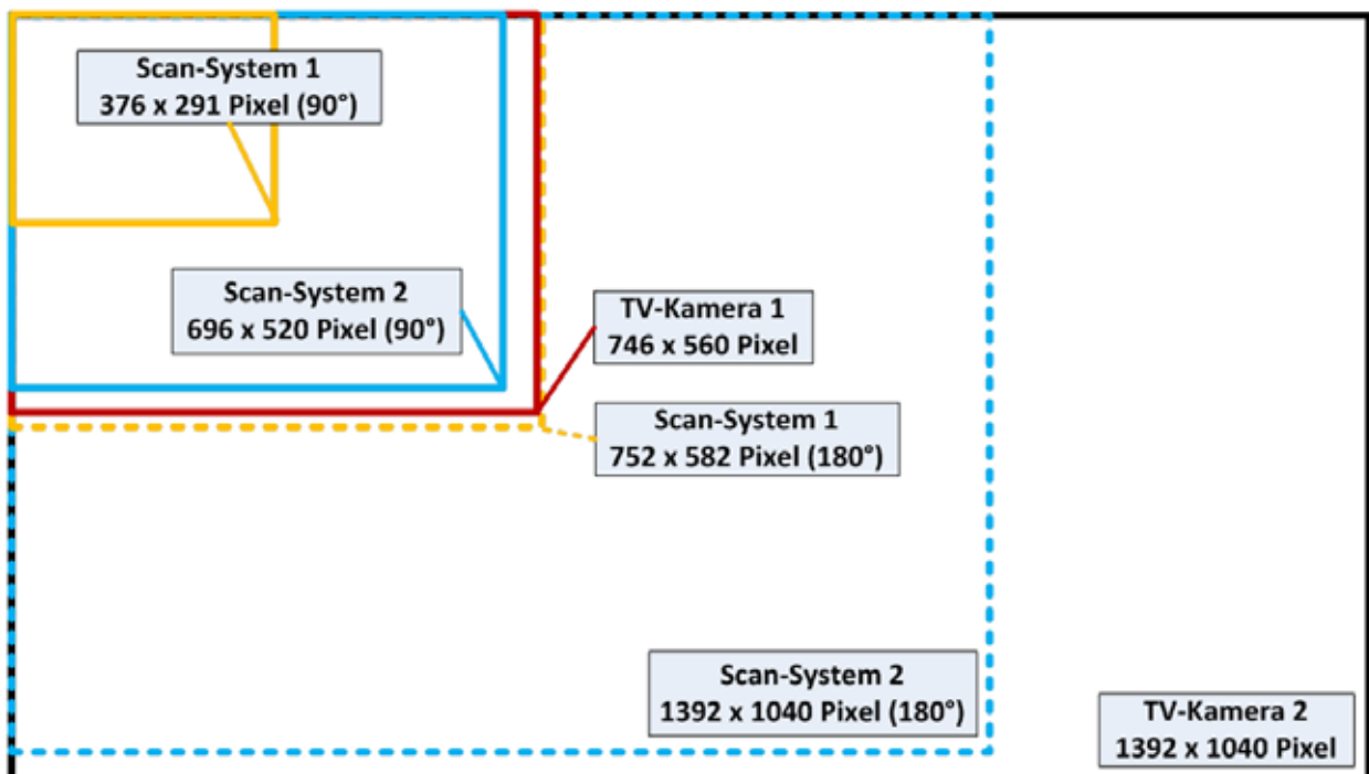
Abbildung 61 - EPC Voruntersuchungen: Vergleich der Bildauflösungen der Inspektionssysteme
