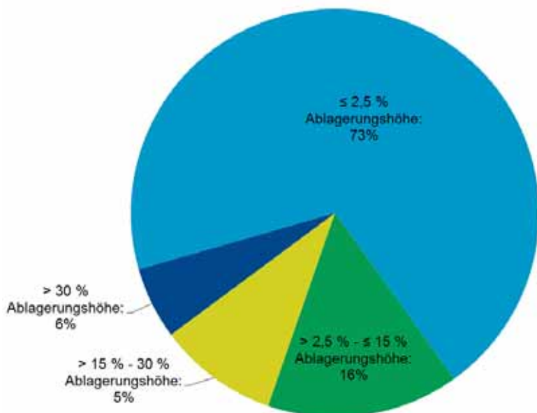
Abbildung 147 - Anteile Ablagerungshöhe in Haltungen der Trennkanalisation
