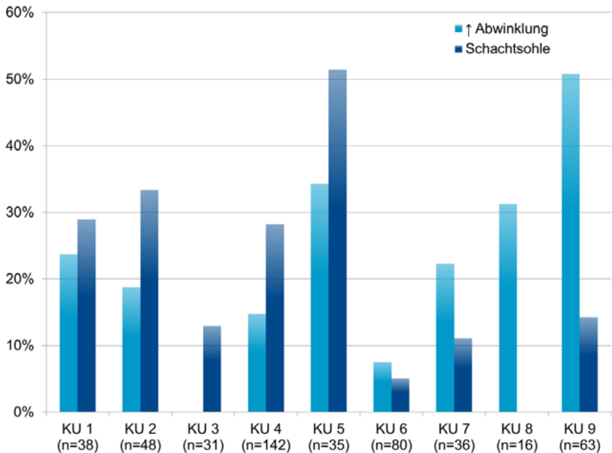
Abbildung 98 - Bauliche Hindernisse je nach Kanalisationsunternehmen (KU)
