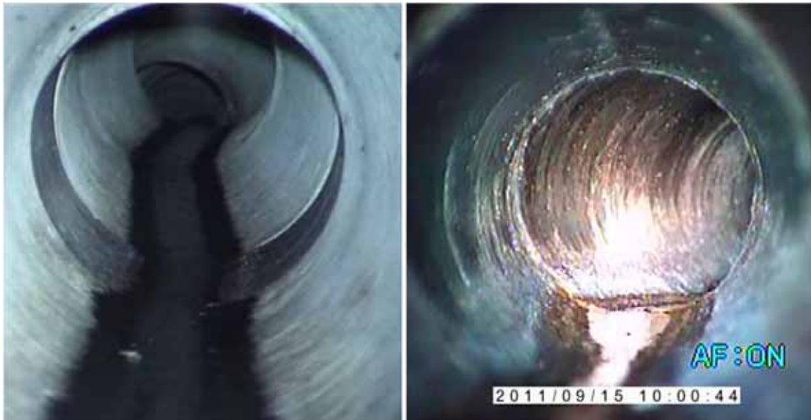
Abbildung 93 - Sicht bis zum Endschacht durch zu große Abwinkelung nicht möglich
