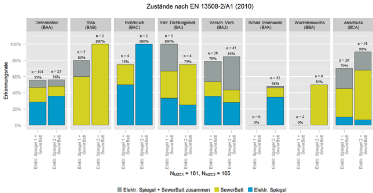
Abbildung 107 - Felduntersuchungen - Kombinierte Erkennungsraten für Spiegelmodell 1 + SewerBatt® und Spiegelmodell 2 + SewerBatt® (Plihal et al, 2015)
