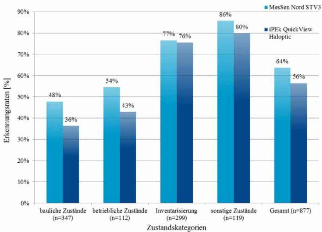
Abbildung 128 - Erfassungsraten elektronischer Spiegel 2011 ohne Zustandsgruppen
