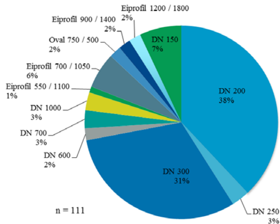
Abbildung 38 - Felduntersuchungen in Kombination Elektronischer Spiegel und SewerBatt® - Haltungsdurchmesser
