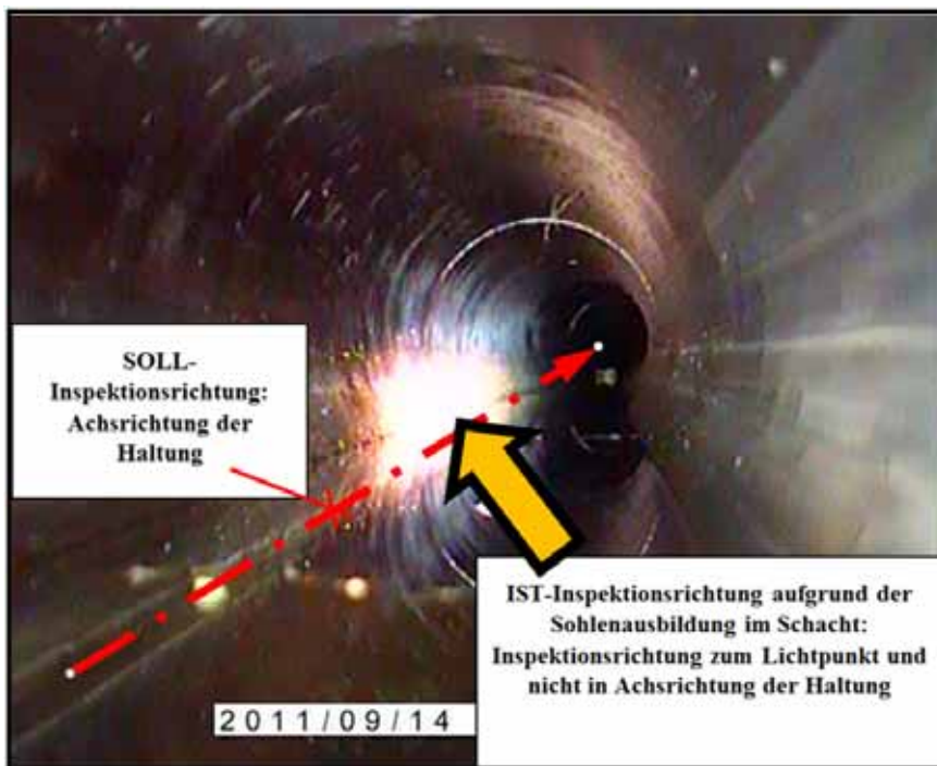
Abbildung 95 - Abweichung der Inspektionsrichtung aufgrund der Sohlensausbildung im Schacht
