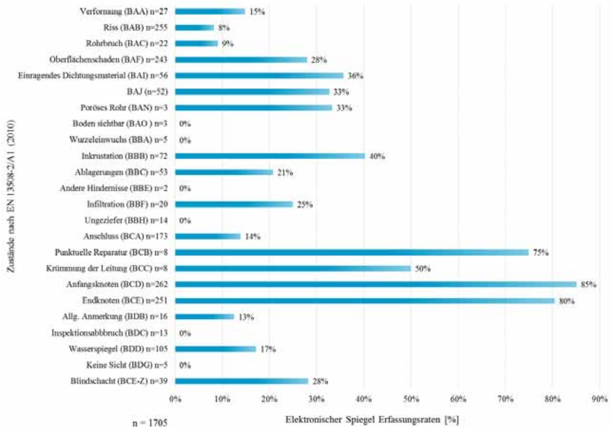
Abbildung 131 - Zustandserfassung der Einzelzustände nach Zustandskodierungen mit elektronischen Spiegel bei Verwendung von Zustandsgruppen 2009/10/12
