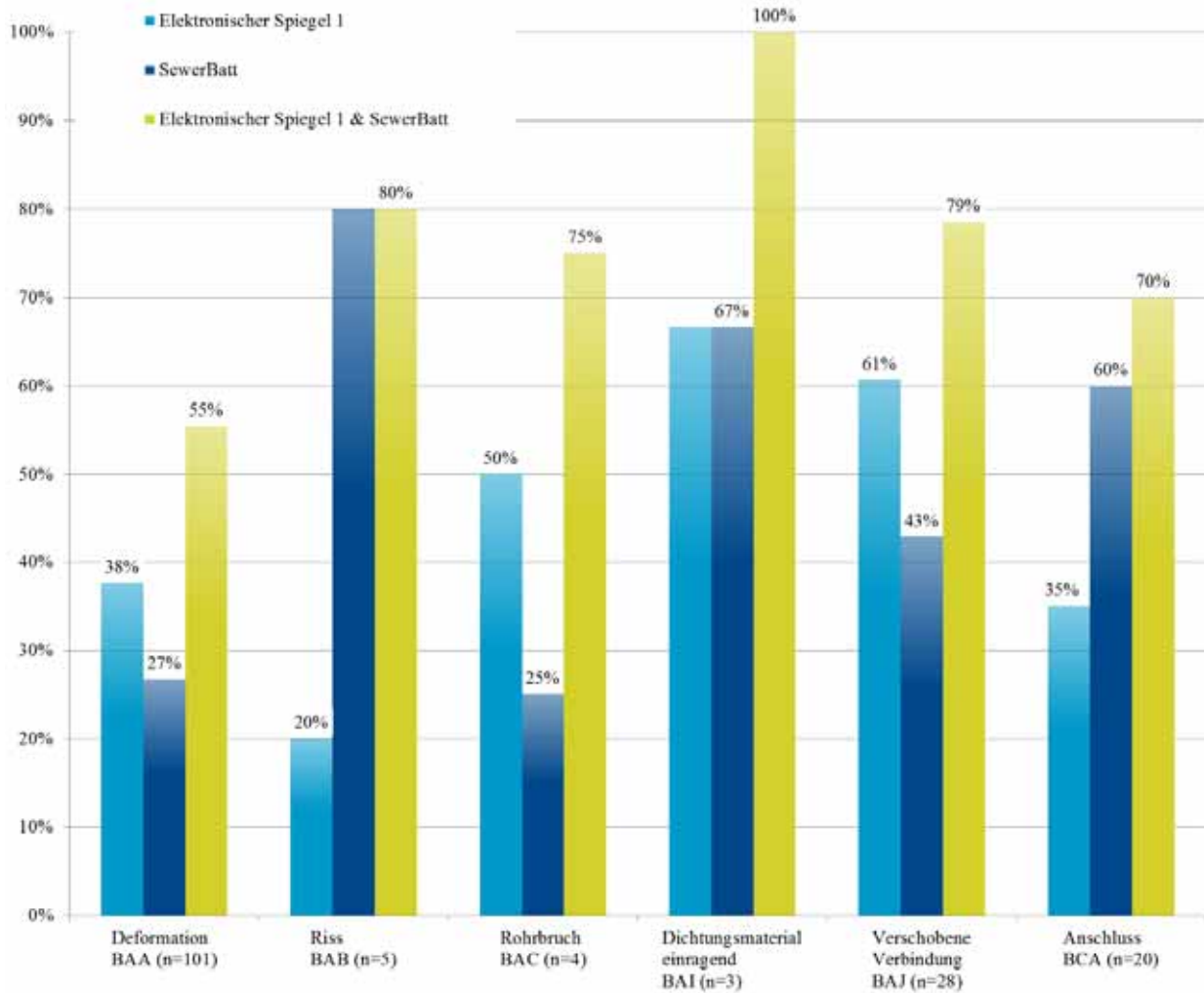
Abbildung 105 - Felduntersuchungen - Individuelle und kombinierte Erkennungsraten für elektronisches Spiegelmodell 1 und SewerBatt® (Plihal et al., 2015)
