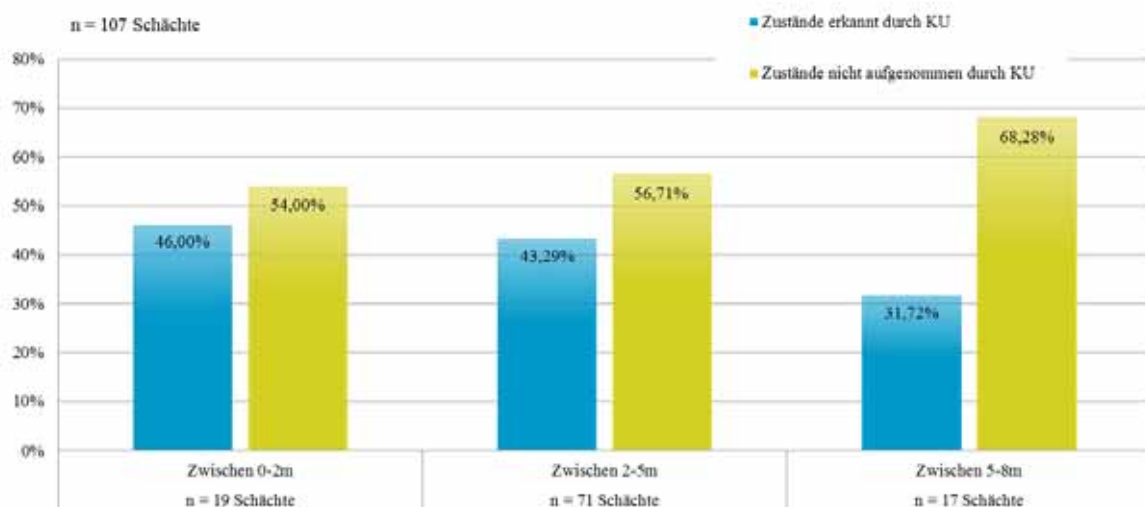
Abbildung 120 - Zustandserfassung in Abhängigkeit der Schachttiefe
