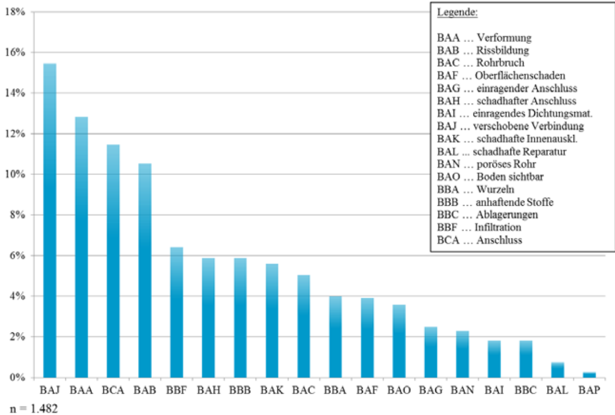
Abbildung 36 - Häufigkeitsverteilung der dokumentierten Zustände
