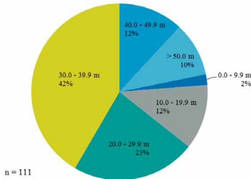
Abbildung 37 - Felduntersuchungen in Kombination Elektronischer Spiegel und SewerBatt® - Haltungslängen
