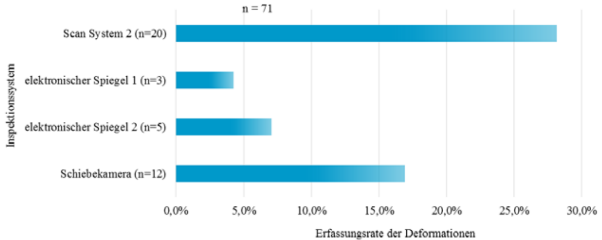
Abbildung 78 - Optische Inspektion: Erfassungsraten von Deformationen (EPC Voruntersuchungen)
