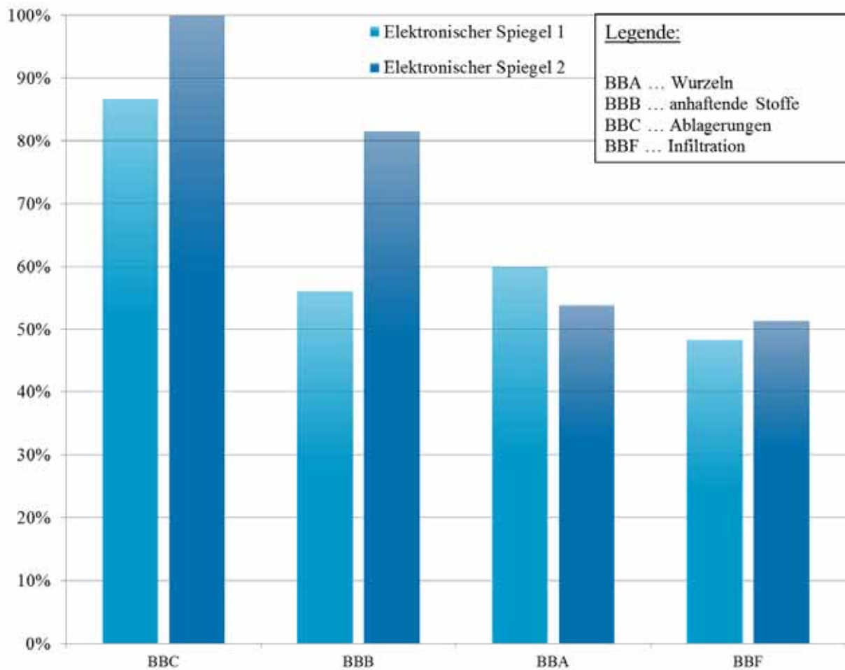
Abbildung 86 - Betriebliche Zustandserkennung in den ersten 15 m beginnend vom Schacht
