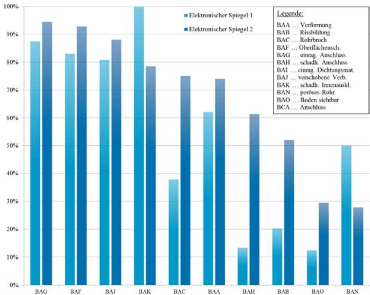
Abbildung 80 - Bauliche Zustandserkennung in den ersten 15 m beginnend vom Schacht
