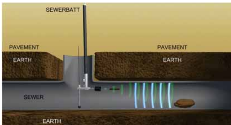
Abbildung 13 - Schematische Darstellung einer akustischen Messung (Horoshenkov, 2013)
