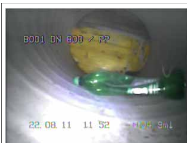
Abbildung 48 - BBE-C: Andere Hindernisse, allgemein; Nennw.-Red.=1%; Kreisprofil DN 800 - Polypropylen; Schiebekamera
