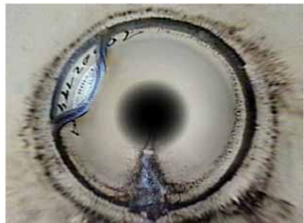
Abbildung 68 - BAI-A-B einragendes Dichtungsmaterial, Dichtring, hängend, nicht gebrochen oberh. Mitte; Kreisprofil DN 200 - Glasfaserverstärkter Kunststoff; Scan System 1
