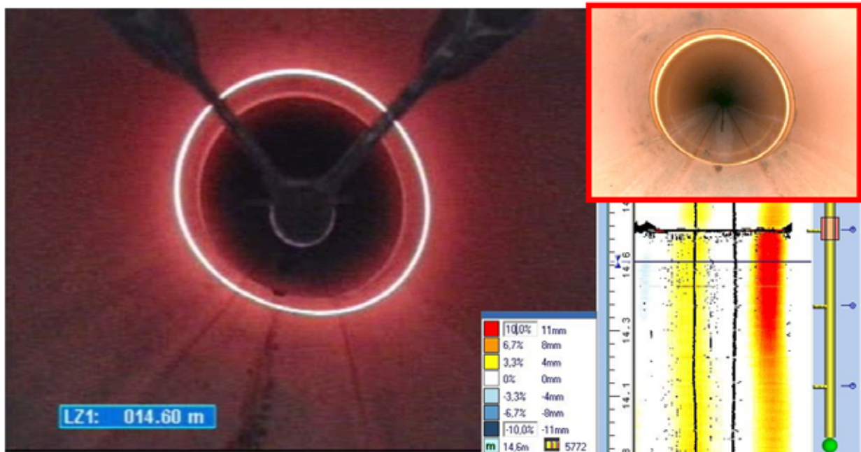
Abbildung 76 - Laser Profiler - Beispiel einer Aufnahme mit 10%iger Deformation (PVC DN 230)
