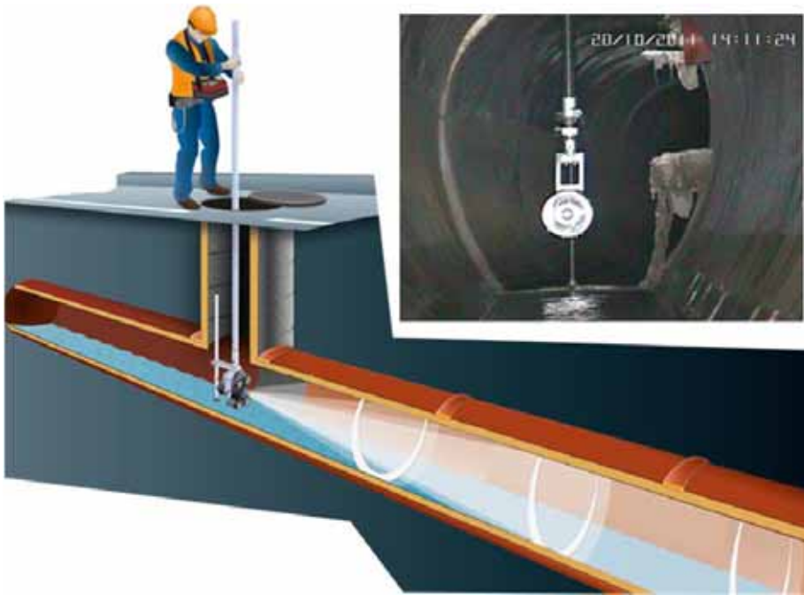
Abbildung 8 - Anwendung eines elektronischen Spiegels (MesSen Nord, 2013 und Plihal et al., 2013a)
