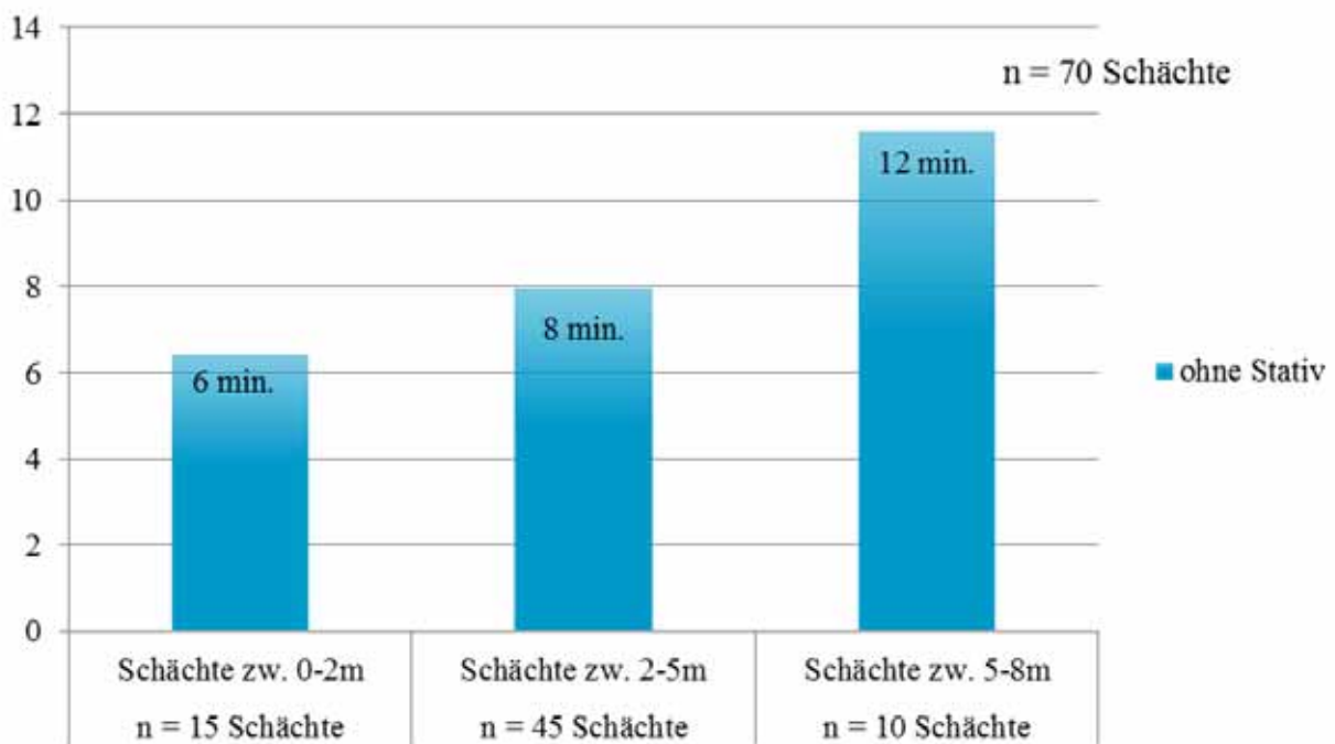
Abbildung 118 - Durchschnittliche Inspektionszeit pro Schacht ohne Stativ
