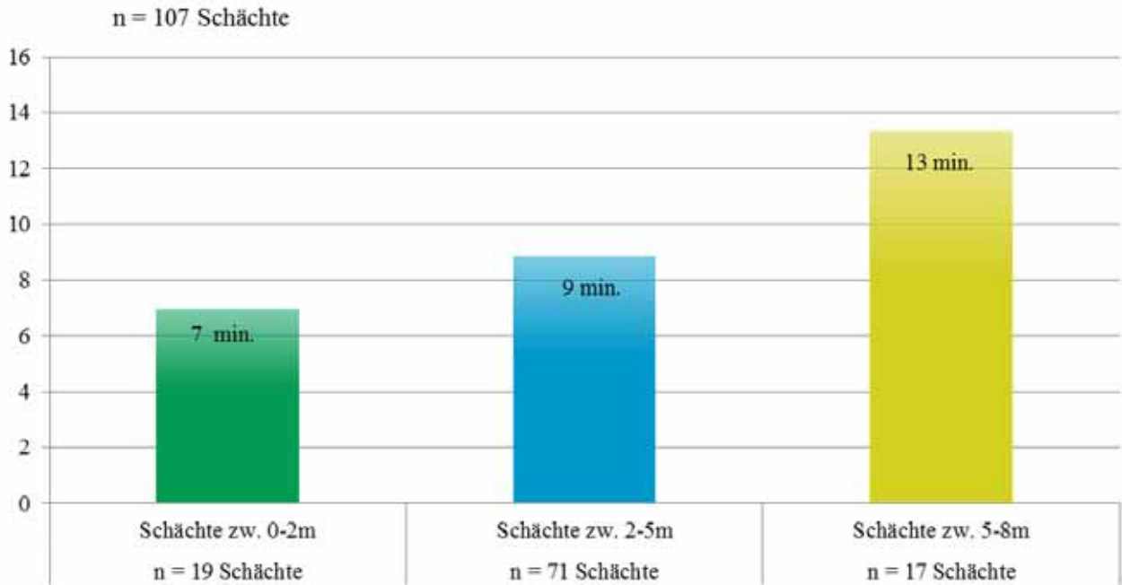
Abbildung 117 - Durchschnittliche Inspektionszeit pro Schacht (mit als auch ohne Stativ)
