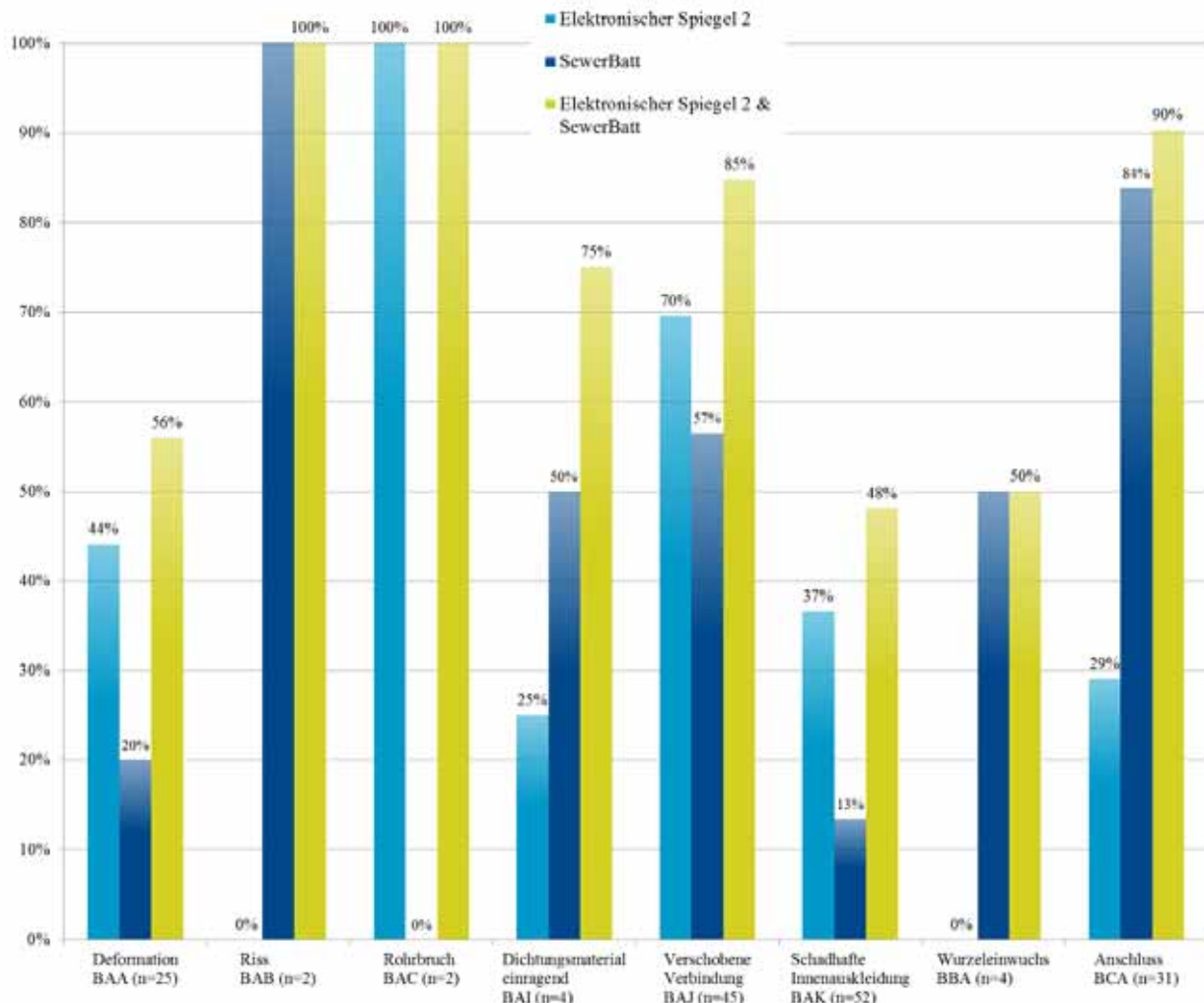
Abbildung 106 - Felduntersuchungen - Individuelle und kombinierte Erkennungsraten für elektronisches Spiegelmodell 2 und SewerBatt® (Plihal et al., 2015)
