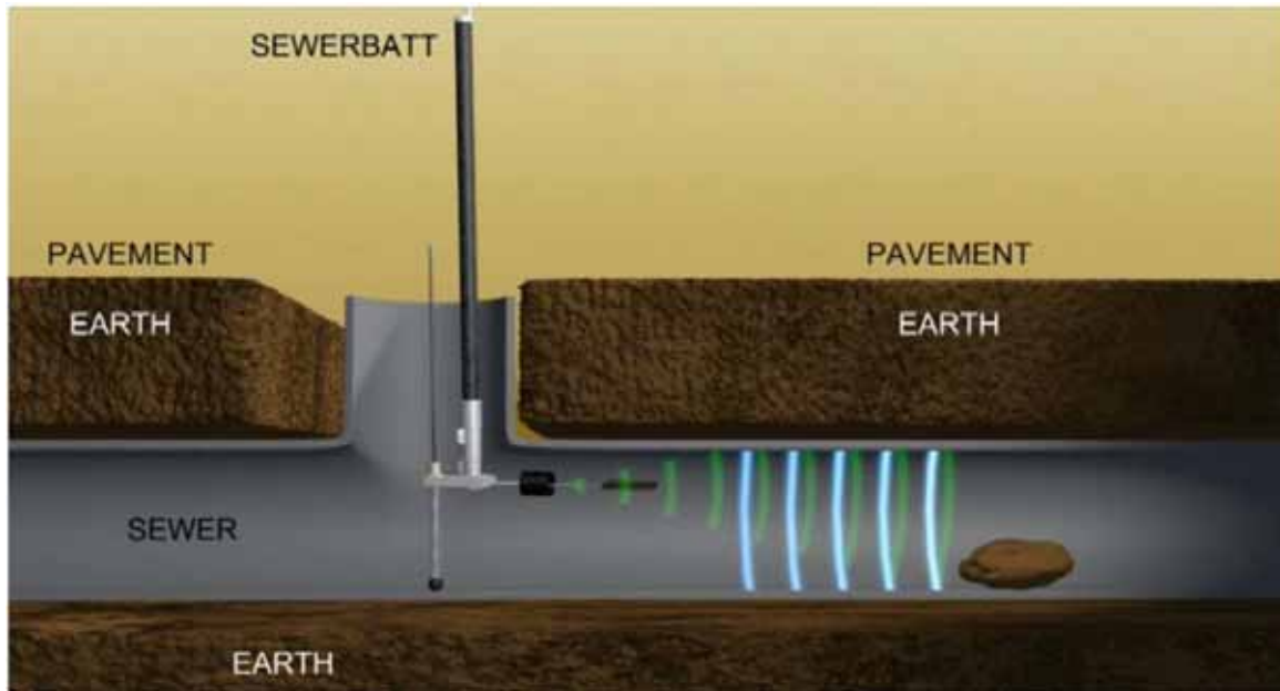
Abbildung 29 - Funktionsweise SewerBatt® (Horoshenkov, 2013)
