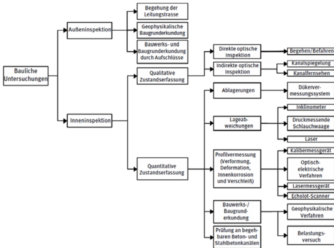
Abbildung 3 - Verfahren zur Untersuchung des baulichen und betrieblichen Zustands von Kanalhaltungen (DWA-M 149-5, 2009)
