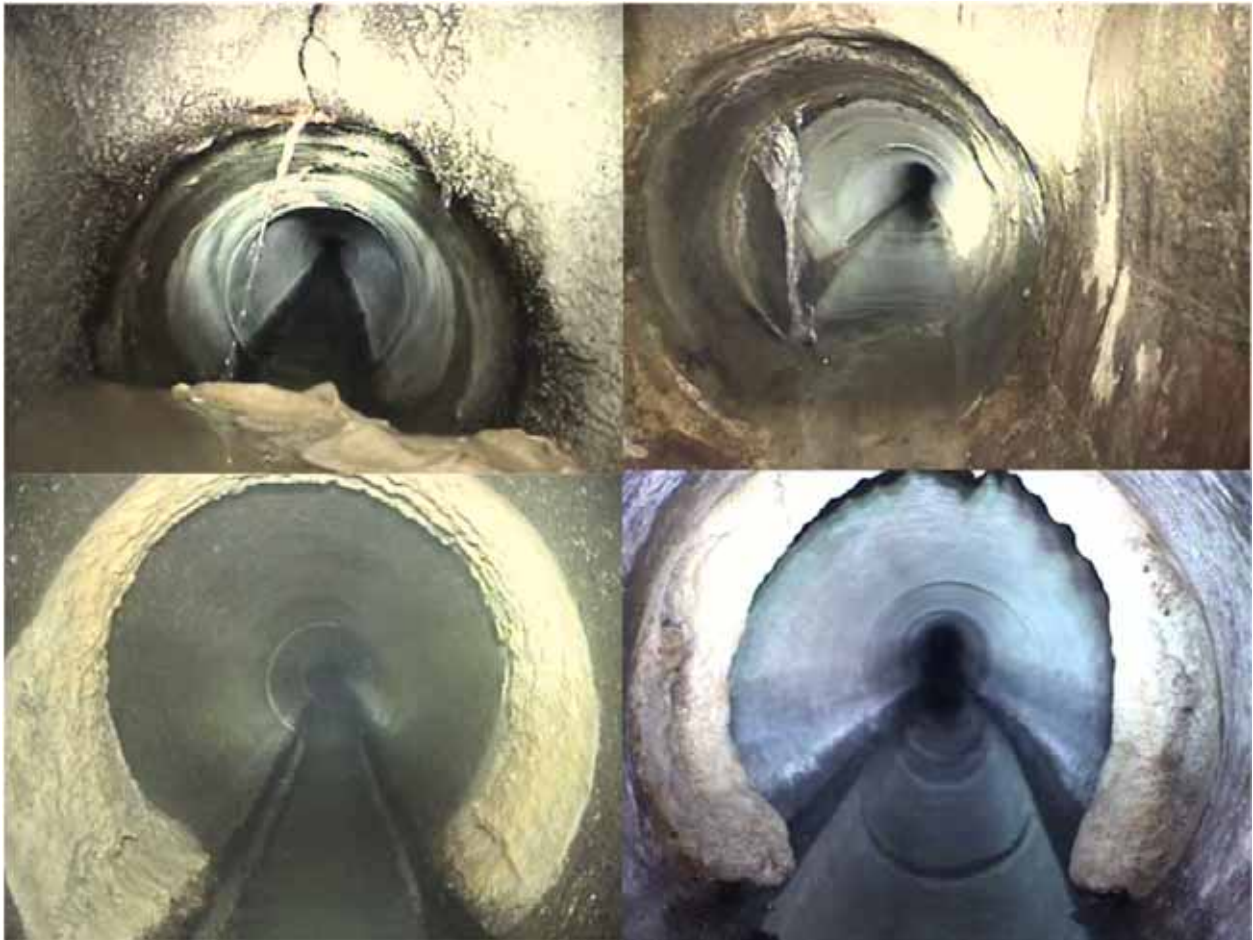
Abbildung 89 - Infiltrationsarten
