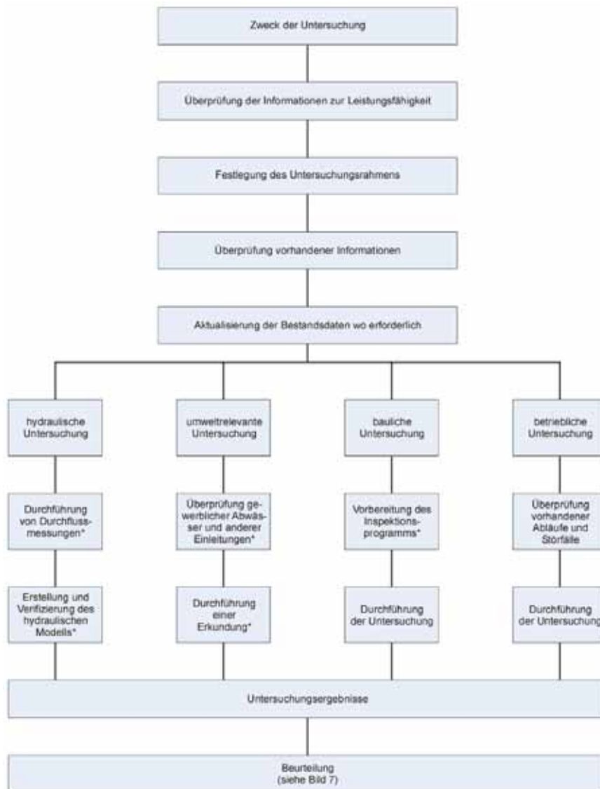
Abbildung 2 - Fließschema von Untersuchungen (ÖNORM EN 752, 2008)
