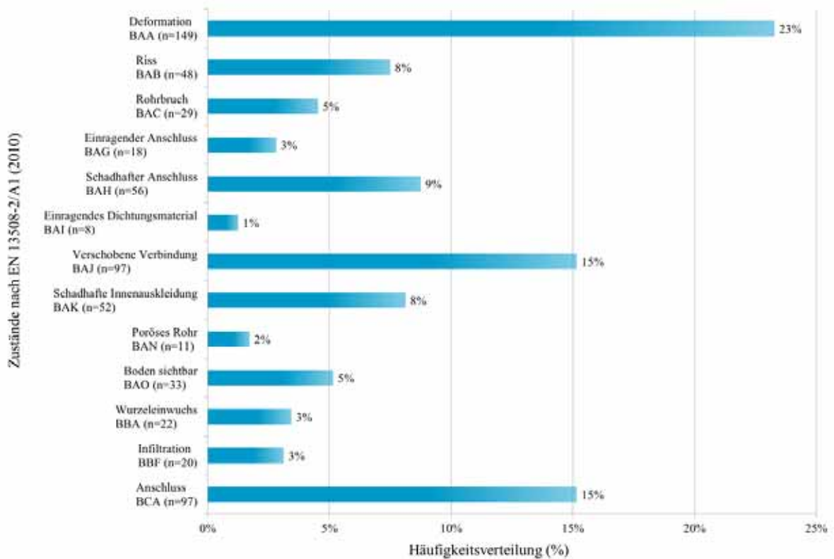
Abbildung 40 - Häufigkeitsverteilung der Zustände der untersuchten Haltungen für die Kombination Elektronischer Spiegel mit SewerBatt®
