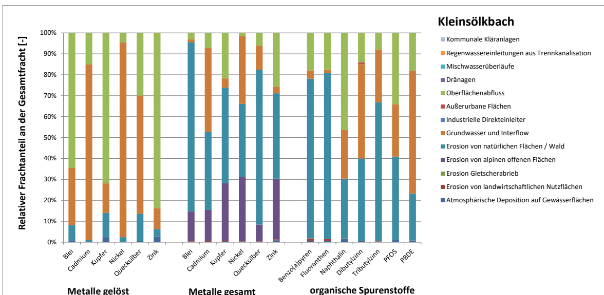
Abbildung 129: Relative Anteile [%] an der Gesamtfracht, die über unterschiedliche Eintragspfade in den Kleinsölkbach eingebracht werden.
