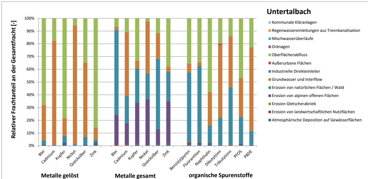
Abbildung 128: Relative Anteile [%] an der Gesamtfracht, die über unterschiedliche Eintragspfade in den Untertalbach eingebracht werden.
