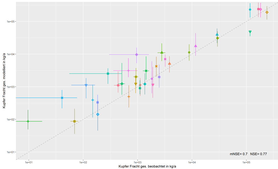
Abbildung 81: Pegelabgleich mit GZÜV-Daten für Kupfer (gesamt).
