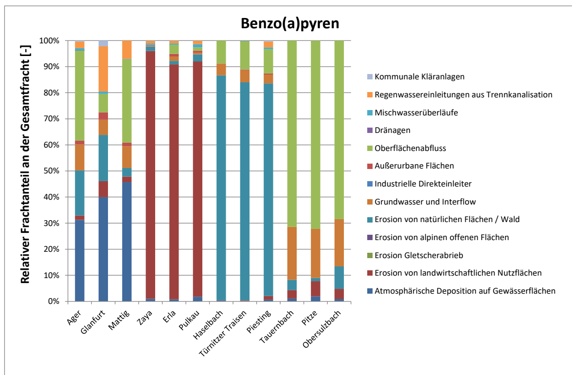
Abbildung 57: Relative Frachtanteile [%] der unterschiedlichen Emissionspfade an der Gesamtemission von Benzo(a)pyren, für exemplarisch ausgewählte Analysegebiete mit den Haupteintragspfaden atmosphärische Deposition, Erosion und Oberflächenabfluss.
