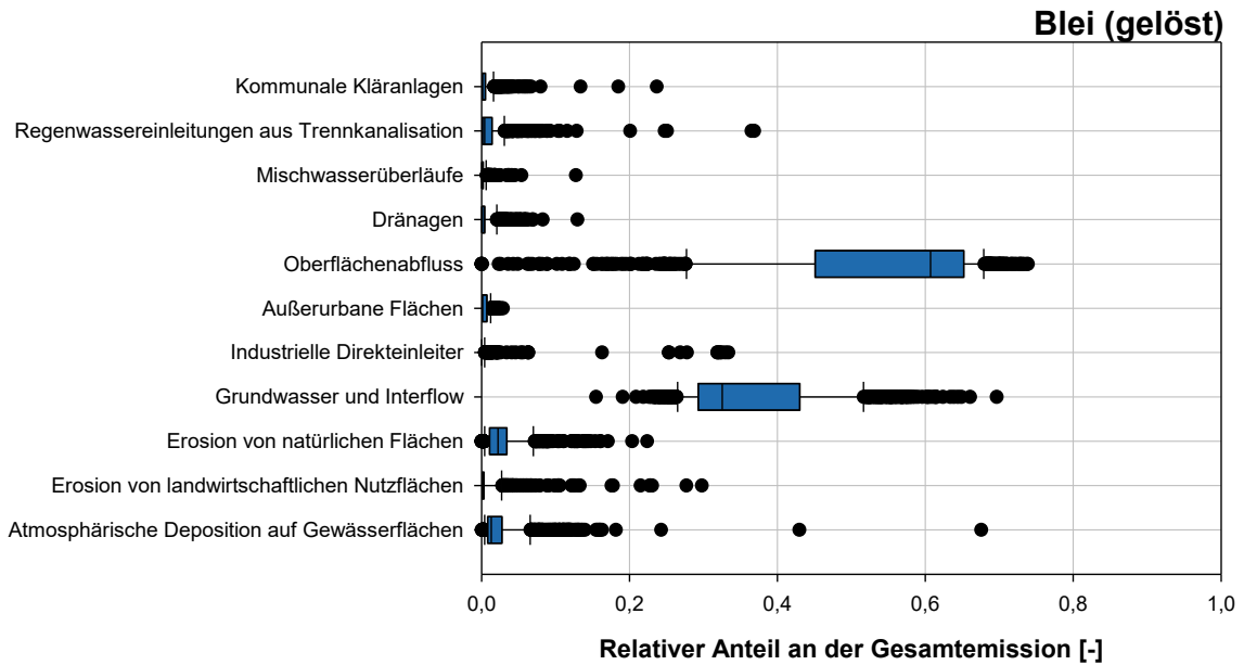
Abbildung 110: Relativer Anteil [-] der unterschiedlichen Eintragspfade in den Gesamteinzugsgebieten der Analysegebiete für Blei (gelöst).
