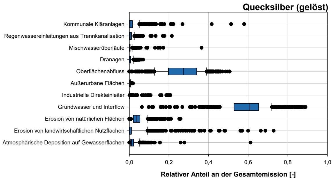
Abbildung 118: Relativer Anteil [-] der unterschiedlichen Eintragspfade in den Gesamteinzugsgebieten der Analysegebiete für Quecksilber (gelöst).
