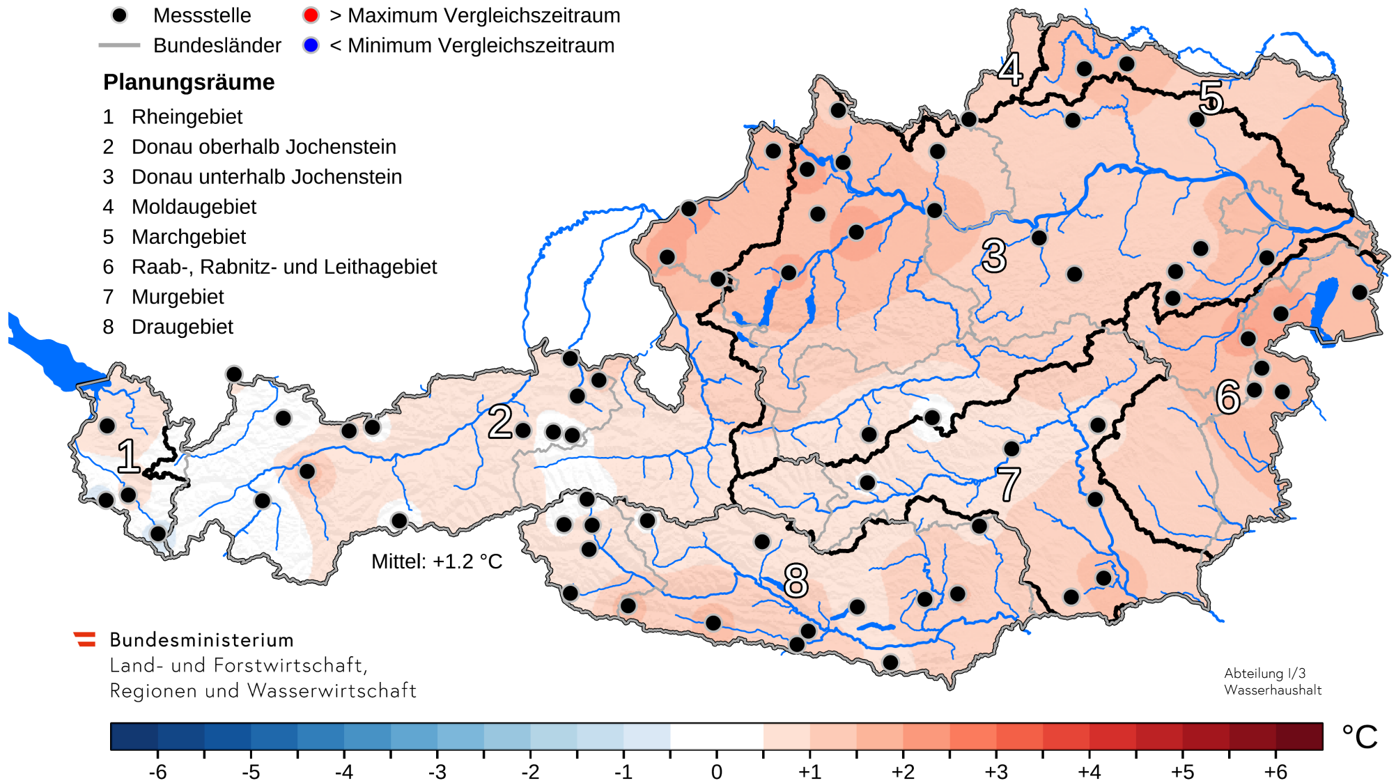
Abbildung 2. Temperaturabweichung in °C des November 2023 vom langjährigen Monatsmittel des Vergleichszeitraums 1981-2010. Rot markierte Messstellen: mittlere Monatstemperatur über dem im Vergleichszeitraum aufgetretenen höchsten Monatsmittel. Blau markierte Messstellen: mittlere Monatstemperatur unter dem im Vergleichszeitraum aufgetretenen niedrigsten Monatsmittel.
