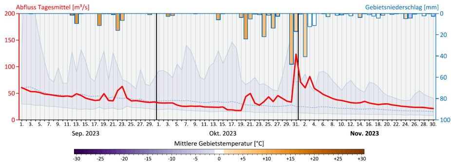
Abbildung 22. Pegel Lienz und Winklarn. Obere Reihe: Abflussganglinien (Tagesmittel) 2023, langjährige Tagesmittelwerte sowie Minima und Maxima der Tagesmittel des Vergleichszeitraums. Untere Reihe: vergangene drei Monate mit zusätzlich dargestellten Tagesgebietsniederschlagssummen (Balken) und mittleren täglichen Gebietstemperaturen (Einfärbung Balken) in den Pegelinzugsgebieten.
