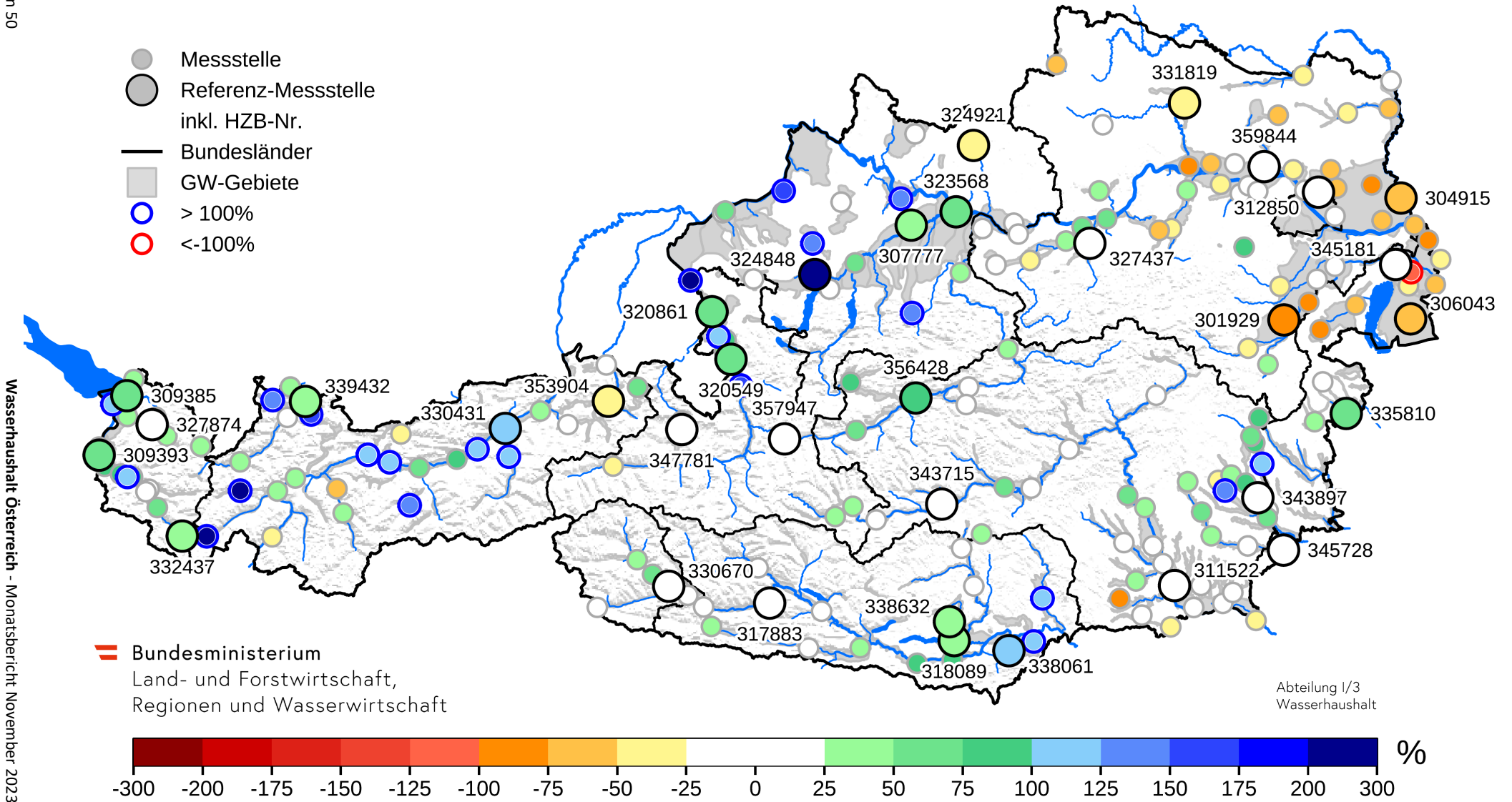
Abbildung 6. Grundwasserstand am letzten Tag des November 2023 im Vergleich zum langjährigen Mittelwert des letzten Tages im November. Ein Wert von 0 entspricht dem langjährigen Mittel, Werte zwischen -100 und 100 entsprechen der im Vergleichszeitraum aufgetretenen Schwankungsbreite. Werte > 100 und < -100 zeigen neue Extrema im negativen und positiven Bereich (zusätzlich blau und rot markiert). Der Vergleichszeitraum zur Ermittlung des langjährigen Mittels variiert an den Messstellen (mindestens zehn Jahre).
