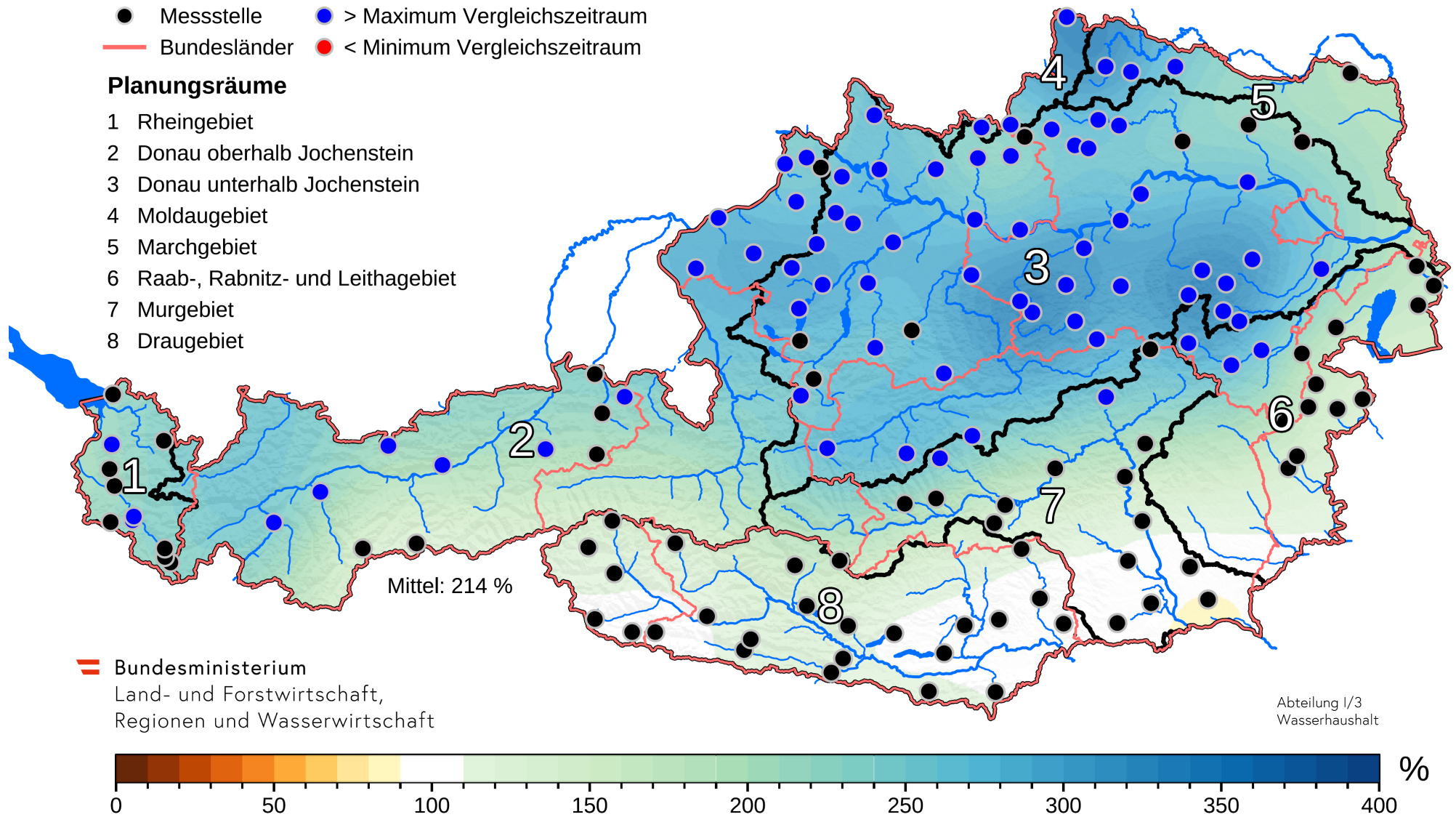
Abbildung 3. Niederschlagssumme des November 2023, ausgedrückt in Prozent der mittleren Niederschlagssumme im November im Vergleichszeitraum 1981-2010. Blau markierte Messstellen: Monatssumme des Niederschlags über der im Vergleichszeitraum aufgetretenen höchsten Monatssumme. Rot markierte Messstellen: Monatssumme des Niederschlags unter der im Vergleichszeitraum aufgetretenen niedrigsten Monatssumme.
