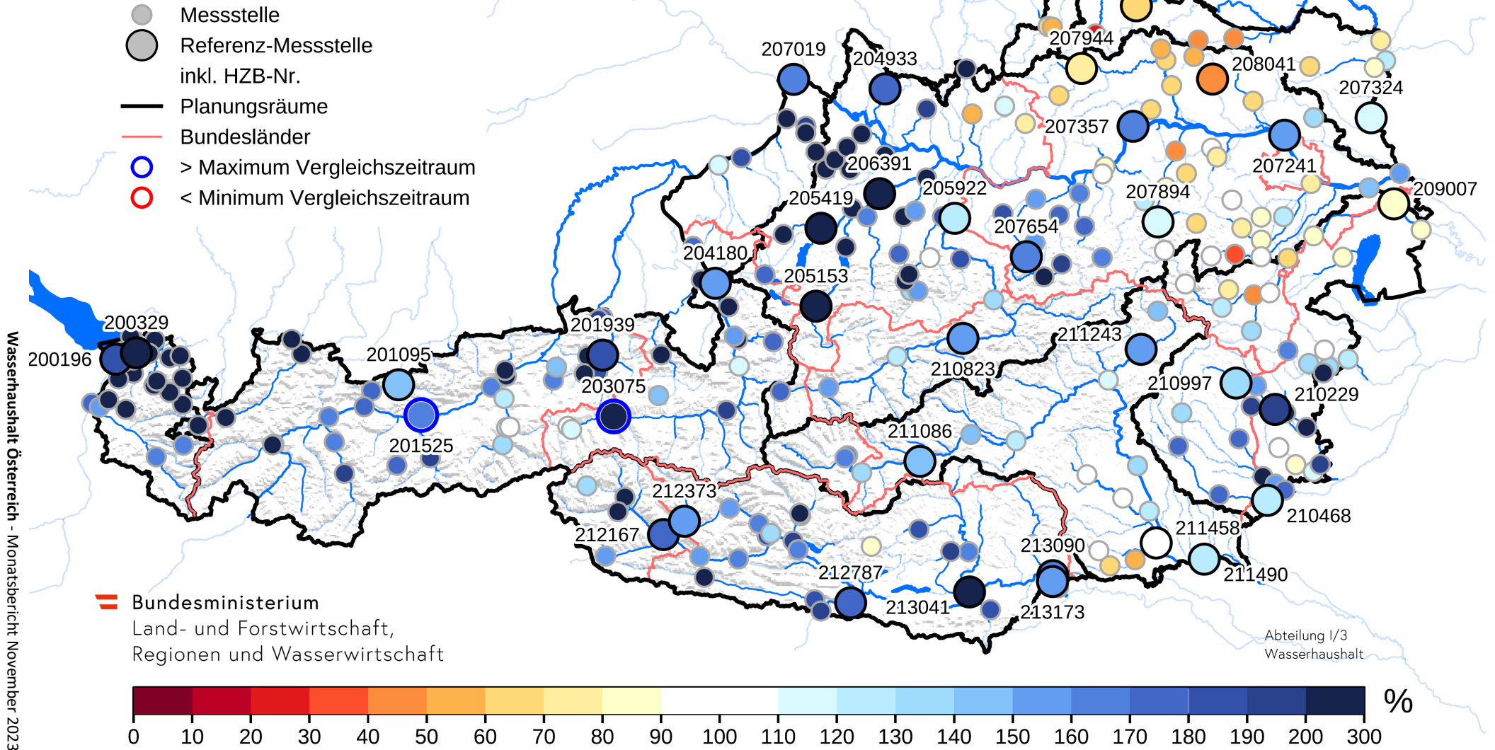
Abbildung 5. Mittlerer Monatsabfluss des November 2023, ausgedrückt in Prozent des langjährigen mittleren Abflusses im November. Ein Wert von 100 entspricht dem langjährigen Monatsmittel. Blau markierte Messstellen: mittlerer Monatsabfluss über dem im Vergleichszeitraum aufgetretenen Maximum. Rot markierte Messstellen: mittlerer Monatsabfluss unter dem im Vergleichszeitraum aufgetretenen Minimum. Der Vergleichszeitraum zur Ermittlung des langjährigen Mittels variiert an den Messstellen (mindestens zehn Jahre).
