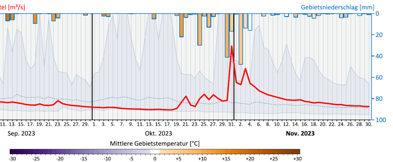
Abbildung 22. Pegel Lienz und Winklarn. Obere Reihe: Abflussganglinien (Tagesmittel) 2023, langjährige Tagesmittelwerte sowie Minima und Maxima der Tagesmittel des Vergleichszeitraums. Untere Reihe: vergangene drei Monate mit zusätzlich dargestellten Tagesgebietsniederschlagssummen (Balken) und mittleren täglichen Gebietstemperaturen (Einfärbung Balken) in den Pegelinzugsgebieten.
