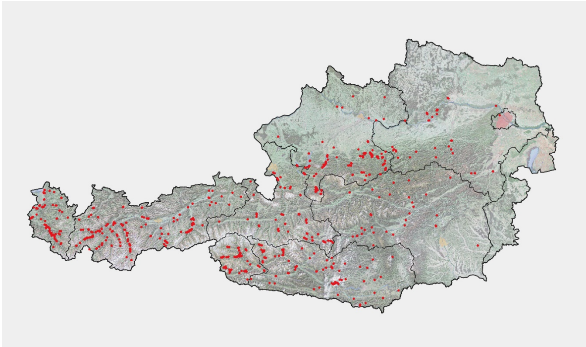
Abbildung 3: Steinschlag-Schutzbauwerke der WLW in Österreich (Auszug aus dem Digitalen Wildbach- und Lawinenkataster, Stand: 12.02.2020)
