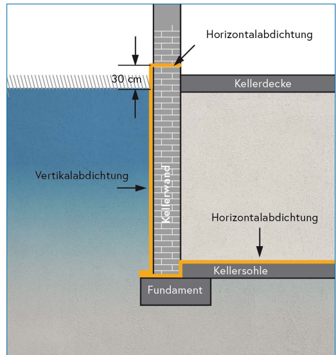
Abbildung 50: Vertikal- und Horizontalabdichtung.
