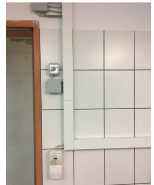
Abbildung 64: In gefährdeten Räumen sollten elektrische Leitungen unbedingt an der Decke verlegt werden. Als Wandverkleidung empfehlen sich Fliesen. Sie erlauben eine einfache und rasche Reinigung nach einem Wasser- oder Schlammeintritt.
