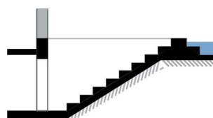
Abbildung 59: Nachträglich durch Aufmauerung geschützter Kellertreppenzugang.
